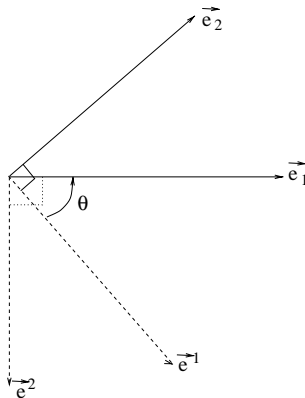
FIG. 2.1 – Base naturelle \vec{e}_i et duale \vec{e}^i
