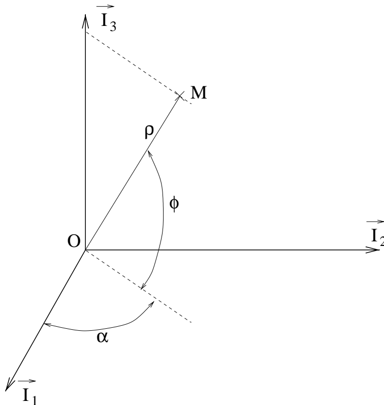
FIG. 6.2 – Systèmes de coordonnées sphériques
