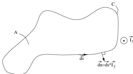
FIG. 6.1 – Cas d'une surface
