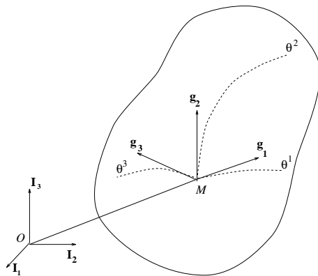
FIG. 4.1 – Définition des vecteurs de base \mathbf{g}_i
