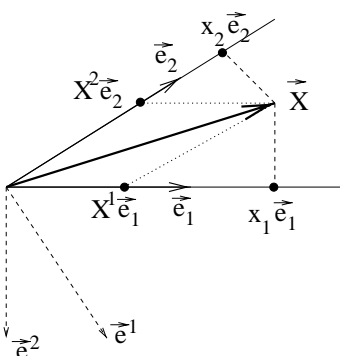
FIG. 2.2 – Composantes covariantes et contravariantes
